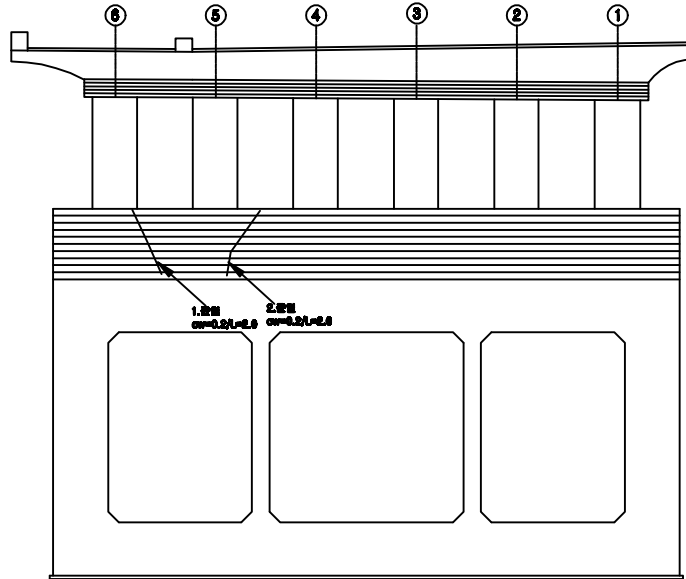
정면도
