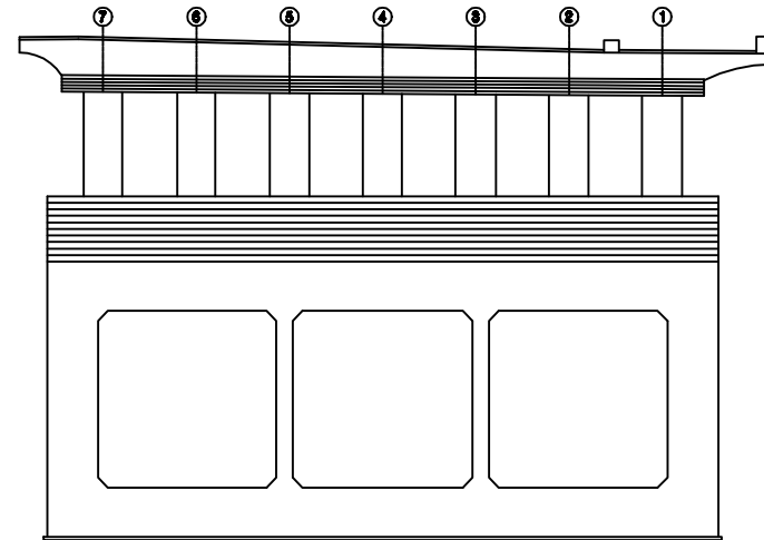
배면도
